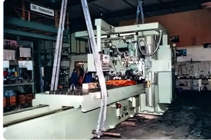
Die Maschine hängt im Kran.
