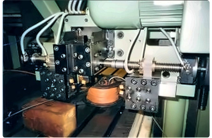
Schlittensystem mit mehreren Stählen im Eingriff.
