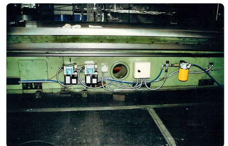
Zusätzliche Schmierung an den Lufteintritten.
