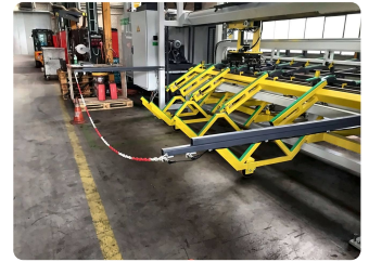
Sicherheitskette vor dem Lichtschrankenbereich.
