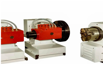
Zwei feststehende Revolver, zwei verfahrbare Spindelstöcke.
