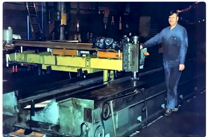
Fräsen der Bettführungen vor Ort. Das Foto ist älter, wir bitten die Bildqualität zu entschuldigen.
