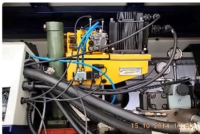
Externe X-Bremse, damit Motoren ohne Bremse genügen.
