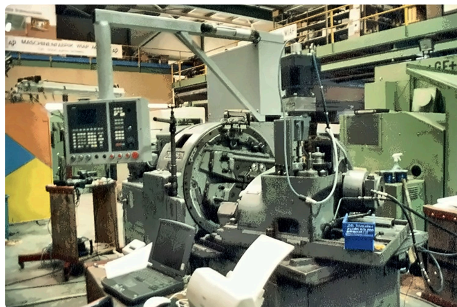
Neu: drei Vorschubmotoren, Elektroschrank kompakt an der Maschine.
