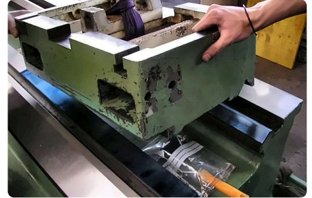
Schlitten beim Abtuchieren.
