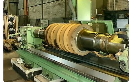
Walzen von mehreren Tonnen Gewicht.
