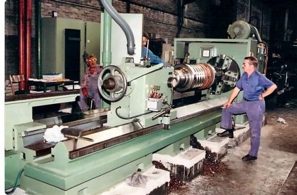
Umgebaute Maschine mit Walze.
