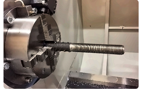
Planspiralfutter: kein Backenwechsel bei anderen Durchmessern.
