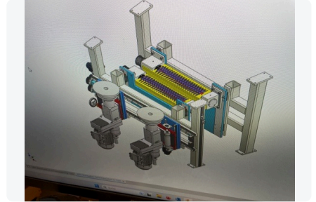
Schlittenträger mit Seitenfräser und Schlitz- und Fassenfräser. CAD
