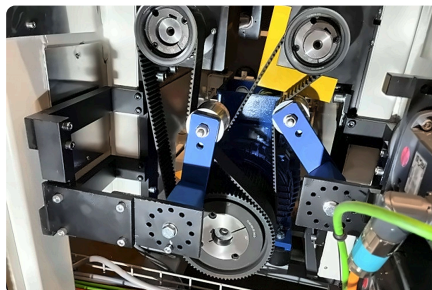
Antrieb des Schlitz- und Fassenfräses.
