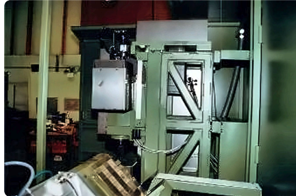
Bettssystem mit Turm, vibrationsentspannt und gedämpft.
