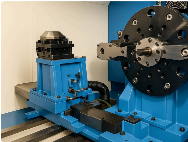
Hinterer Kopfrevolver auf eigenem Schlitten.
