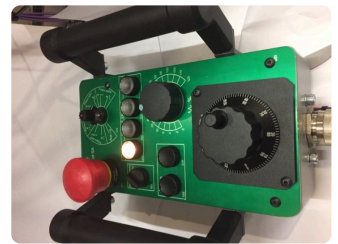
WIAP-Handrad mit Notstopp.
