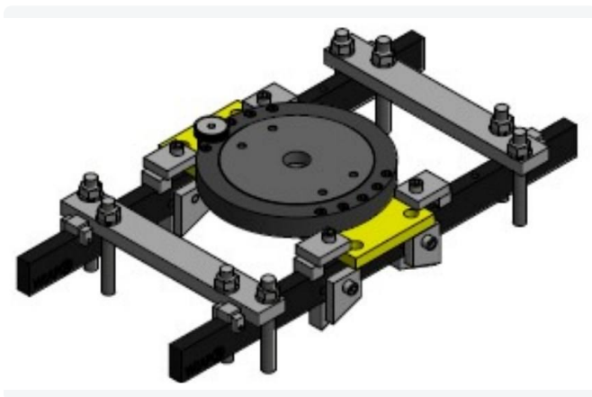
Aufspannvorrichtung für Rundteile (Konstruktionsmodell): Spann- und Drehvorrichtung als Basis eines Mehrachs-Vibriersystems.
